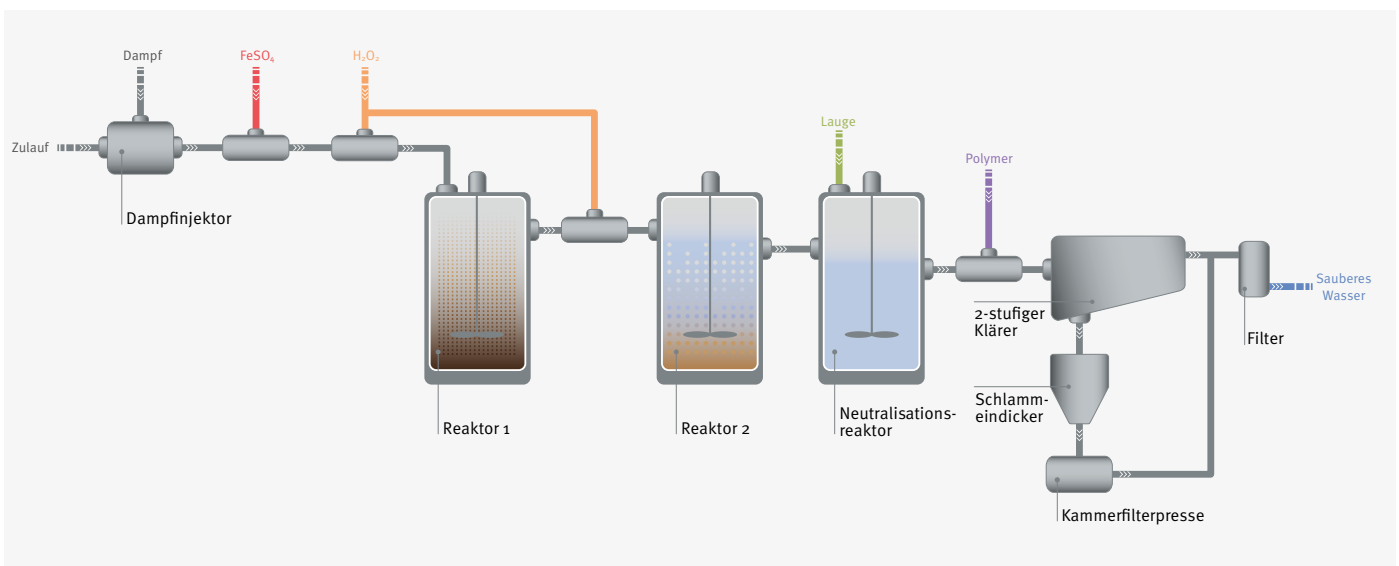
Übersicht des Fentox-Prozesses.
